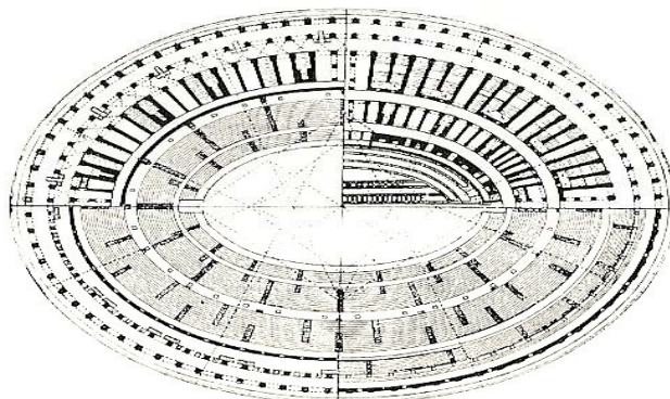
c) Flavio o Colosseo (Roma) 80 d. C. asse maggiore m. 187,75 asse minore m. 155,60 capienza spettatori 102.000 circa
