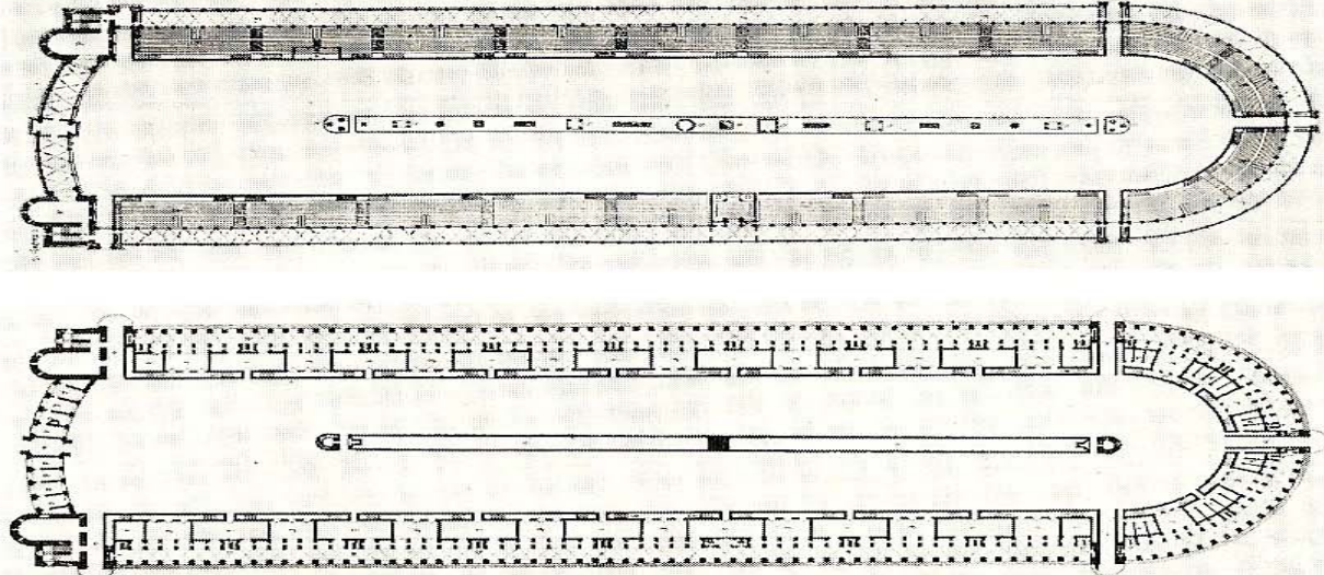
Fig. 37 - Circo detto di Gaio e Nerone costruito in Roma da Caligola nel I secolo d. C. asse maggiore m. 350 asse minore m. 100 capienza spettatori 23.000 circa a) piante (scala 1:3500) b) ricostruzione prospettica.
