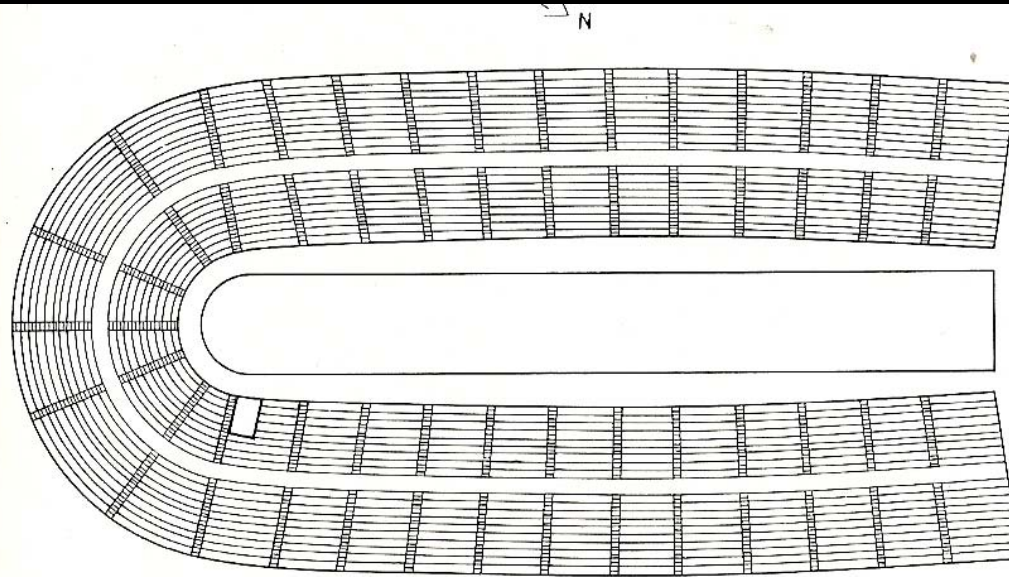
Fig. 25 - Atene: Stadio Panatenaico restaurato. asse maggiore m. 255 asse minore m. 131 capienza spettatori 50.000 circa Costruito da Erode Attico nel II secolo d.C., semidistrutto nelle epoche seguenti, fu restaura- to per la munificenza del greco Giorgio Averoff e riaperto il 24 marzo 1896 con la cerimonia inaugurale della I Olimpiade moderna. a) pianta (scala 1 : 2500) b-c) vedute dello Stadio allo stato attuale. Si noti come nella foto c la folla si disponga nel modo osservato da Gavin Hadden.
