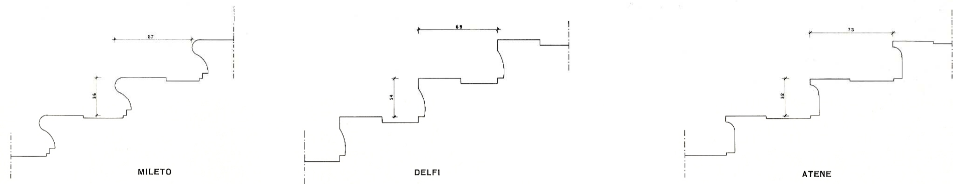
Fig. 23 - Sezioni dei gradoni degli stadi greci di Mileto, Delfi, Atene.
