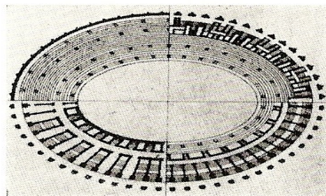
e) Nîmes (Francia) II secolo d. C. asse maggiore m. 140,60 asse minore m. 112,50 capienza spettatori 30.000 circa
